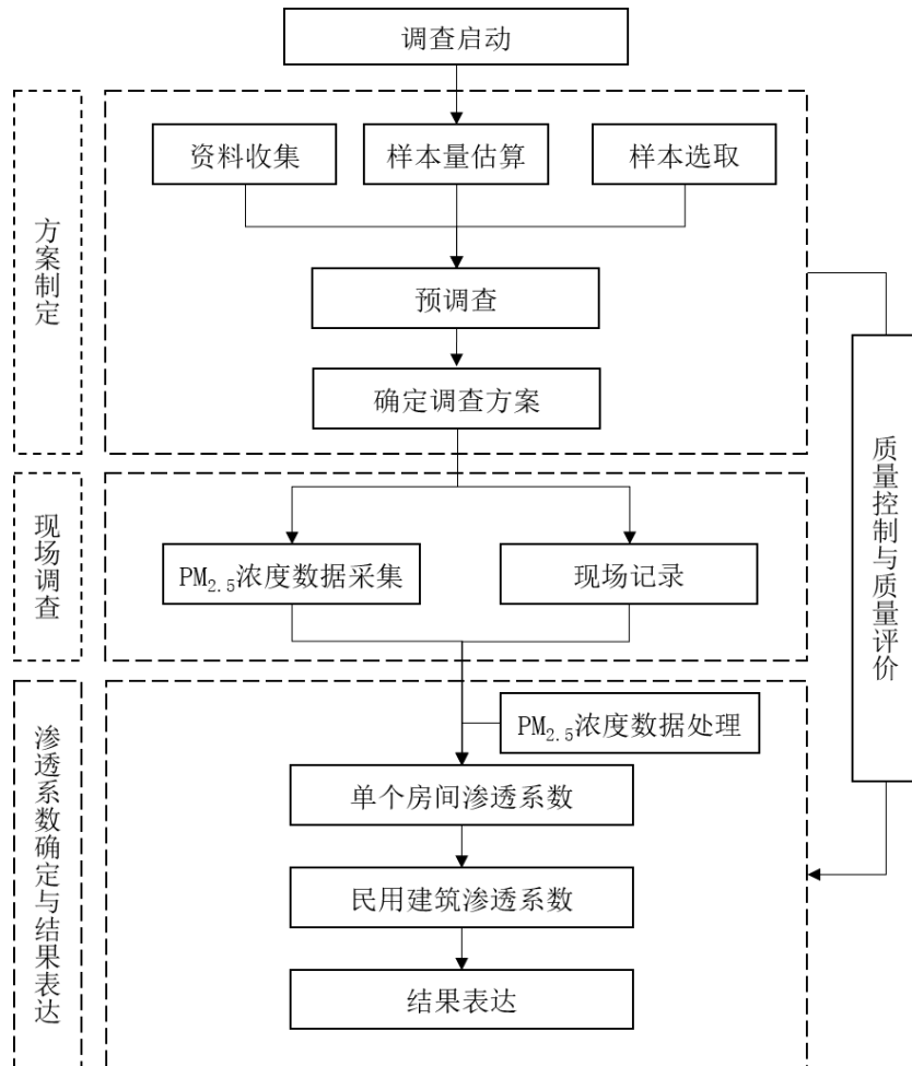
图1 工作程序
